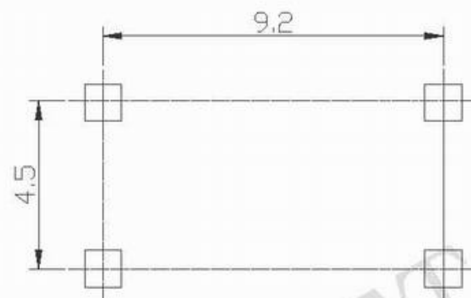
P.C.B. LAYOUT
